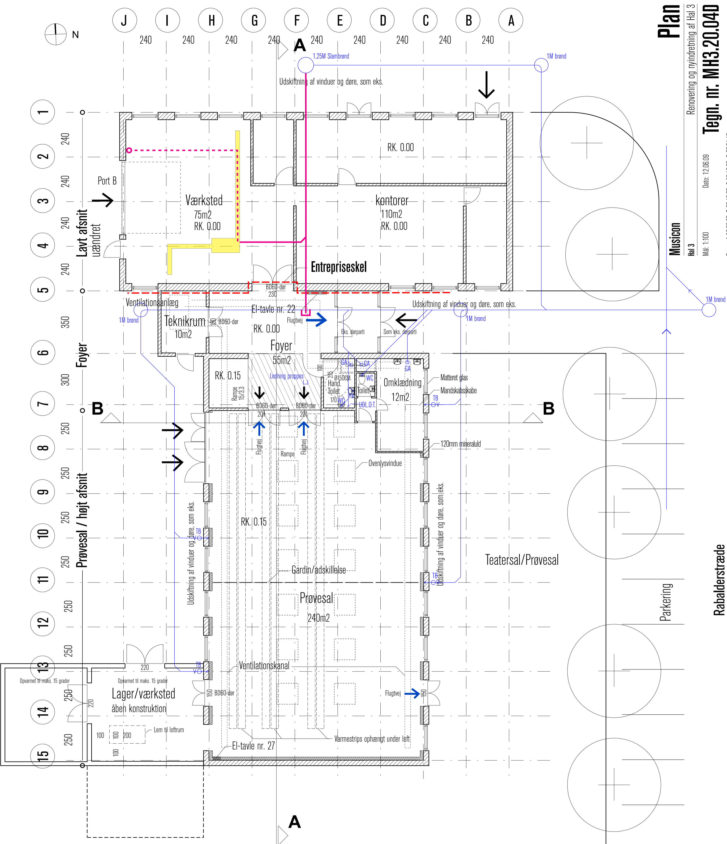
Plan 1:100
